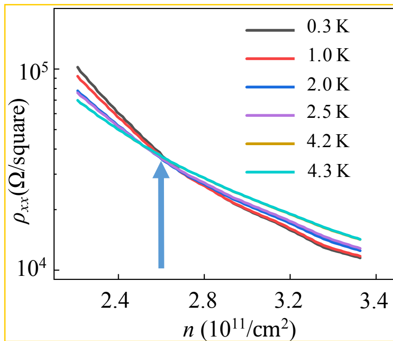
图 4.7 不同温度条件下，零磁场下纵向电阻率随电子浓度的变化关系图。
