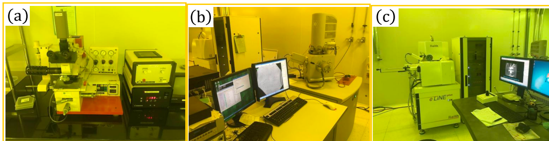
图 2.1 光刻加工设备: (a) SuSS MJB3 型紫外光刻机。(b) 配备了纳米图形生成系统的扫描电子显微镜 FEI Inspect F50, 可以进行电子束曝光。(c) 用于电子束曝光的 Raith E-line plus。
