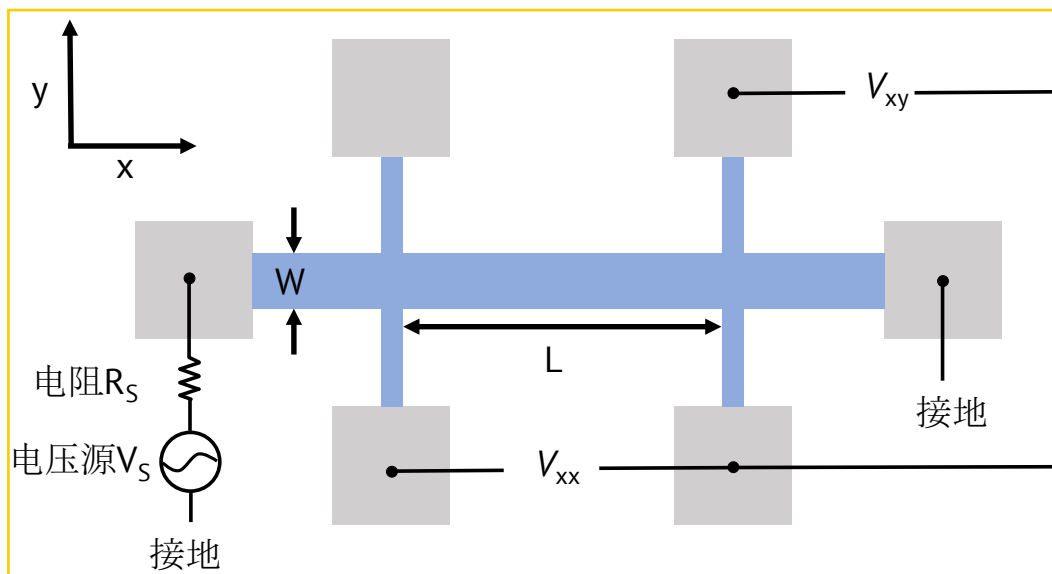
图 2.6 霍尔棒的基本结构和四端法线路连接。线路中 x 方向的直流是通过在欧姆接触一端添加电压偏置产生的，电压源和欧姆接触连接之间会增加一个 10\text{ M}\Omega 或者 100\text{ M}\Omega 的电阻 R_s 来保证电流的稳定性。非掺杂型霍尔棒内部的电阻由顶栅控制，需要保证它远小于 R_s ，这样才能使整个线路基本上工作在恒流状态。需要测量的两个主要参数是 x 方向电势差 V_{xx} 和 y 方向的电势差 V_{xy} 。在测量量子霍尔效应的过程中，会在垂直于器件的 z 方向外加一个磁场。测量区域的尺寸分别用长度 ( L ) 和宽度 ( W ) 表示。
