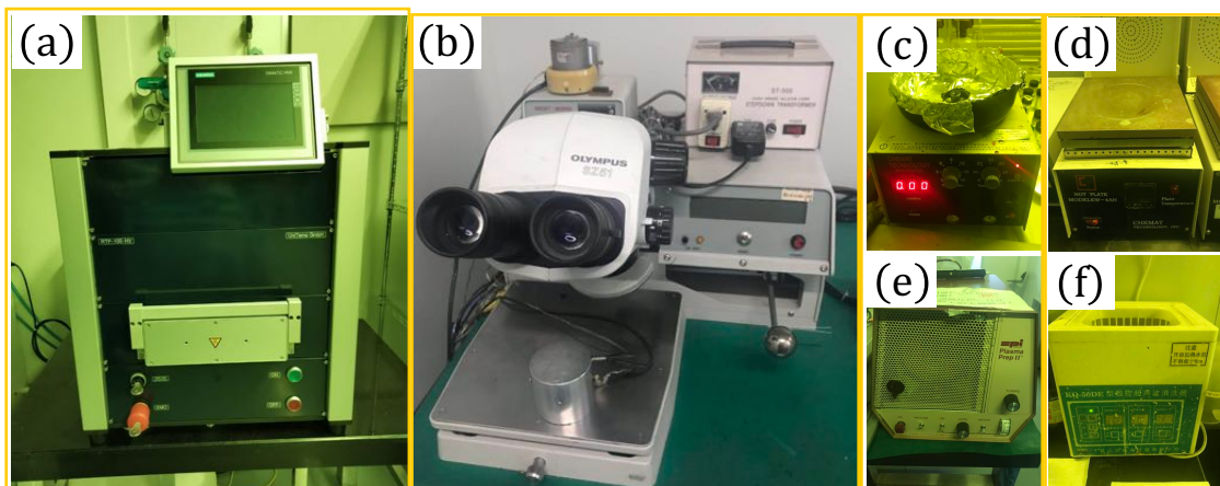
图 2.2 我们实验室使用的其他设备：(a) 退火炉。(b) 键合机。(c) 匀胶机。(d) 加热板。(e) 等离子清洗机。(f) KO-50DE 型超声仪。
