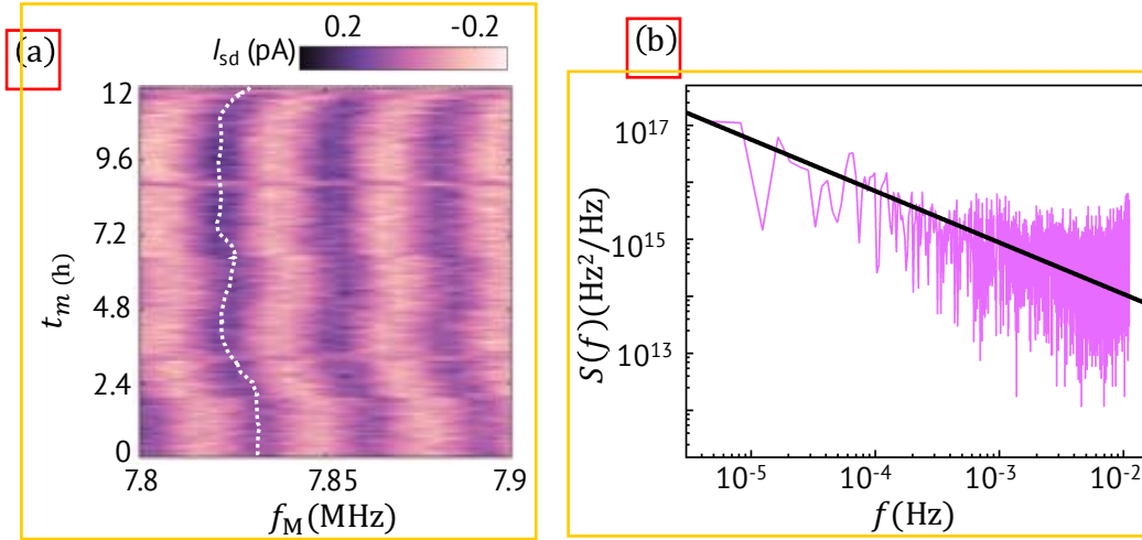
图 5.14 (a) 测量自旋处于激发态随外加微波频率的变化，总的测量时间为 t_m = 121 。所选的自由演化时间为 30\text{ ns} ，从虚线位置提取数据进行参数拟合。(b) 噪声谱随频率的变化关系，基本满足 1/f^{0.9} 的线性。从虚线数据到噪声谱的过程采用 S(f_k) = \frac{t_d}{N} \sum_{n=1}^N |v(t_n) e^{-2\pi i f_k t_n}|^2 。 t_d 是采样间隔， N 是采样点数。
