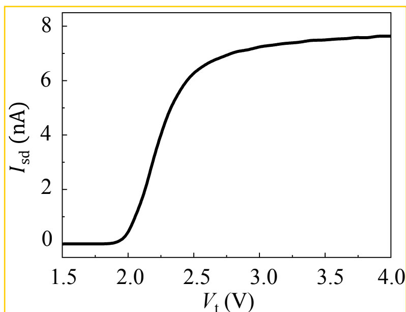
图 4.4 4.2 K 下两端法直接测量电流电压关系。外加的偏置电压为 20 \mu V。
