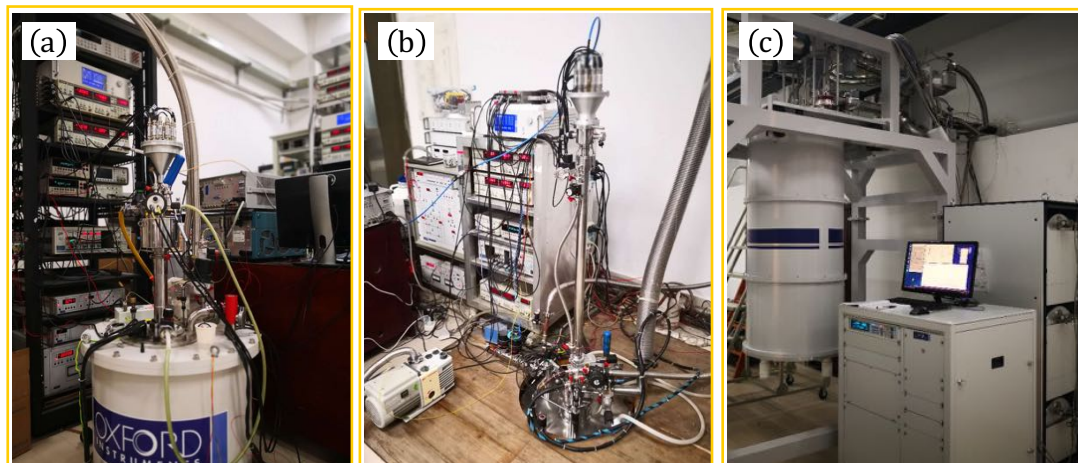
图 2.5 稀释制冷机 (a) He-3 稀释制冷机。(b) Top-loading 式 He-3/He-4 稀释制冷机。(c) 无液氦稀释制冷机。
