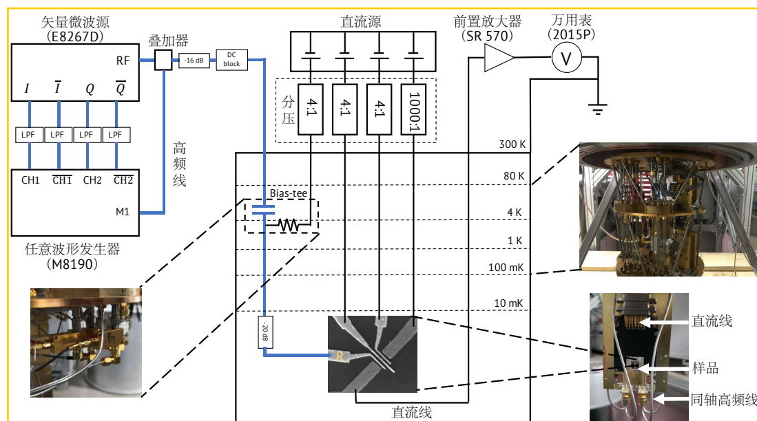
图 2.8 量子比特线路连接以及无液氦稀释制冷机内部主要器件。
