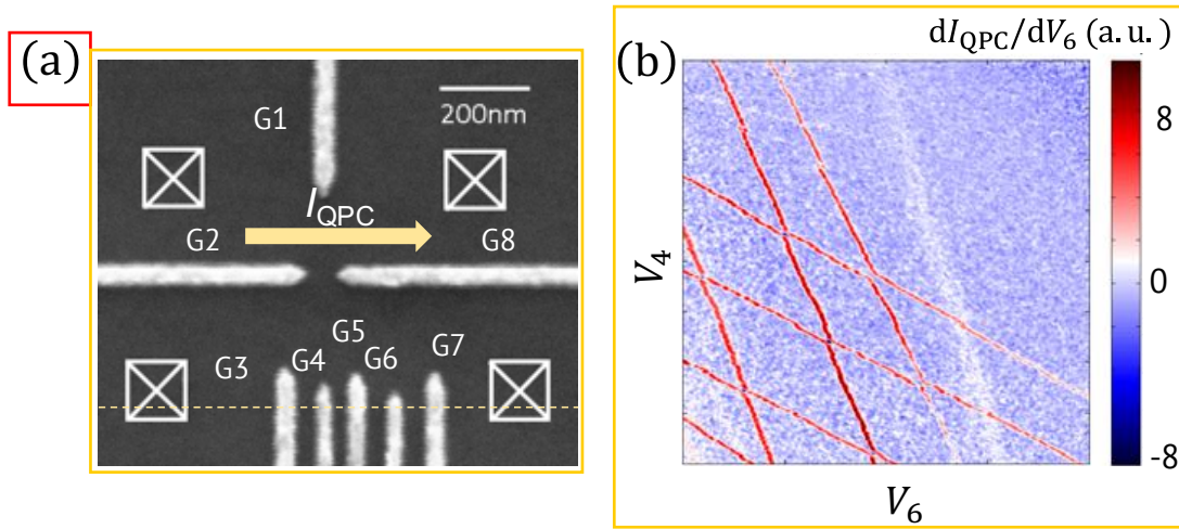
图 3.4 (a) 空穴型 GaAs 双量子点结构。(b) 使用电荷感应技术得到的电荷稳态图。测量的是 QPC 通道中电流 I_{QPC} 的微分电导 dI_{QPC}/dV_6 ，此时交流激励添加在 G6 上，白色带叉方块代表欧姆接触。
