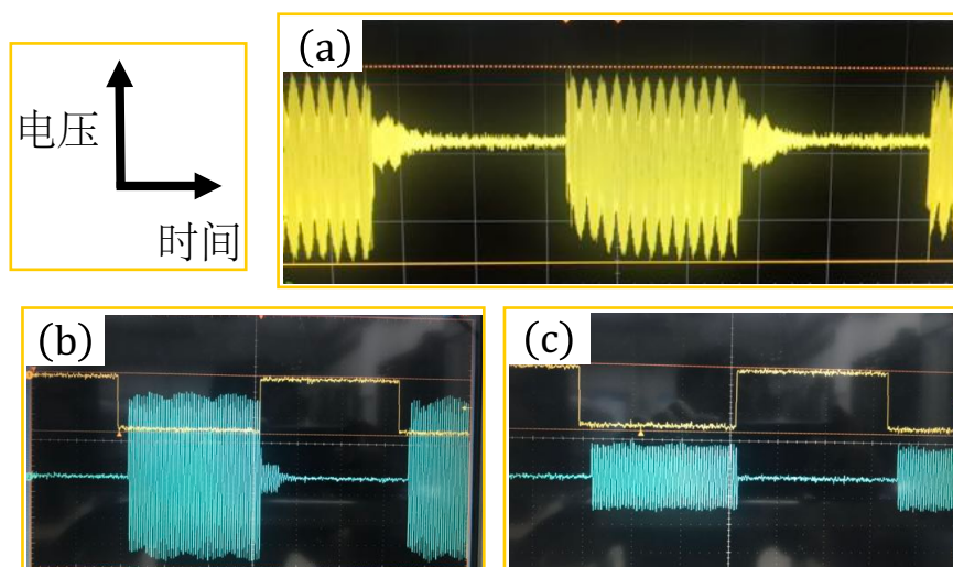
图 2.10 混频后的时域信号 (a) 直接混频, 不进行任何参数优化时结果。(b) 进行 IQ 本征泄漏压制后的信号。(c) 在各个连接处添加 3 dB 的衰减器后结果。
