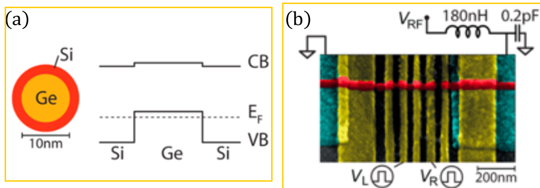
图 5.1 核壳型锗硅纳米线双量子点。(a) 结构与能级。(b) 样品制备成双量子点器件后的实物图。图片引自 [4]
