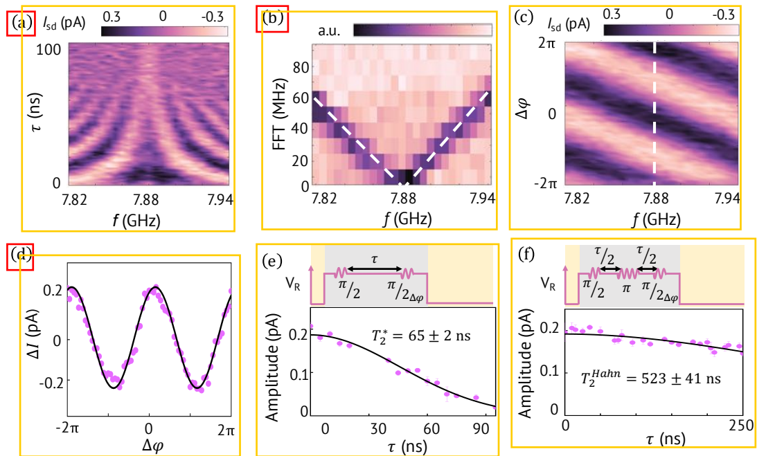
图 5.6 B 模式下（外磁场为 156 mT）的 Ramsey 和 Hahn 回波实验。(a) 不同频率下绕 z 轴自由演化的 Ramsey 振荡。微波功率为 0 dBm，外磁场为 156 mT。对图 (a) 中的演化时间进行傅立叶变换后的实验结果，虚线标注了振荡频率随着失谐频率的变化值，满足 f_{\text{Ramsey}} = f_{\text{MW}} - f_0 。(c) 改变第二个 \pi/2 的相位测得的振荡现象，满足以 2\pi 为周期的振荡。(d) 在微波频率为 7.88 GHz、功率为 0 dB 下的相位控制信号。利用该数据提取振幅，可以较为精确地拟合退相干时间。(e) 按照 (d) 图中的方法提取幅值，幅值随演化时间在减小的过程对应着退相干过程。依据公式 I = A \exp(-(\frac{\tau}{T_2^*})^2) 提取退相干时间 T_2^* 。(f) 进行动力学解耦后的 Hahn 回波测量，依据公式 I = A \exp(-(\frac{\tau}{T_2^{\text{Hahn}}})^{1+\alpha}) 提取 T_2^{\text{Hahn}} ( \alpha = 0.9 ，具体见补充材料)，有效延长退相干时间。以上实验过程中所有的 \pi/2 脉冲为 2.5 ns， \pi 脉冲为 5 ns。
