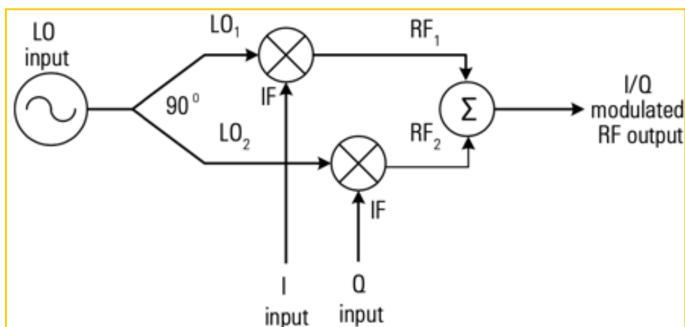
图 2.9 四端口 I/Q 混频器原理图
