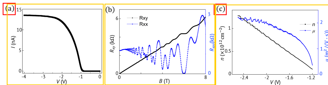
图 2.7 (a) 在外加 20\text{ }\mu\text{V} 交流激励时，不同顶栅电压下回路中的总电流。(b) 顶栅电压为 -2\text{ V} 时，不同磁场下的纵向电阻 R_{xx} = V_{xx}/I 和横向电阻 R_{xy} = V_{xy}/I 。(c) 通过 R_{xx} = V_{xx}/I 和 R_{xy} = V_{xy}/I 计算所得的不同顶栅电压下的空穴态浓度和迁移率。
